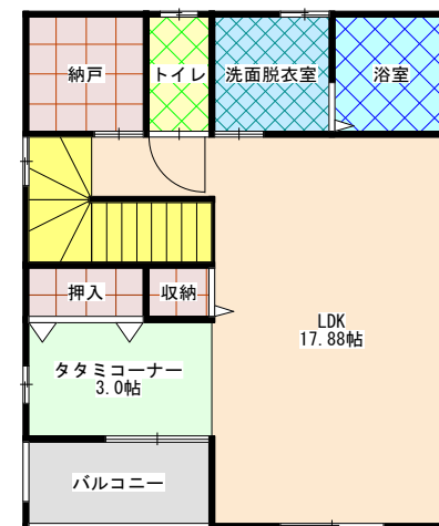
2階平面図
