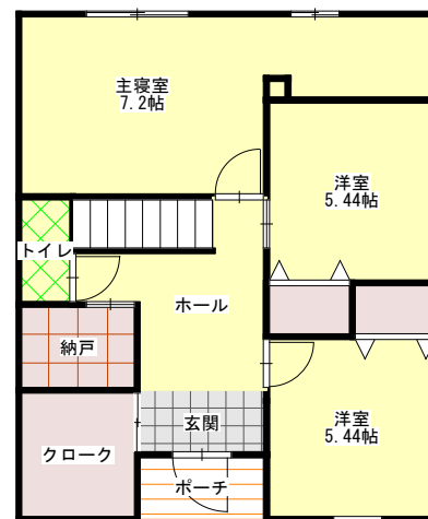
1階平面図
